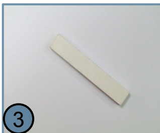
3 Притирка для подгонки щеток 20x12x120мм – предназначена для притирки угольных щеток
